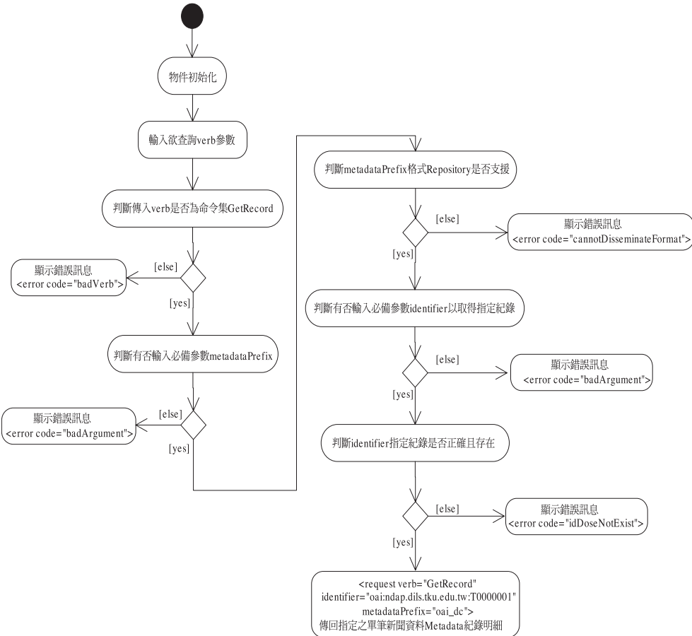
圖9 GetRecords活動圖 (資料來源：本研究繪製)
