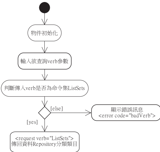
圖6 ListSets活動圖 (資料來源：本研究繪製)
