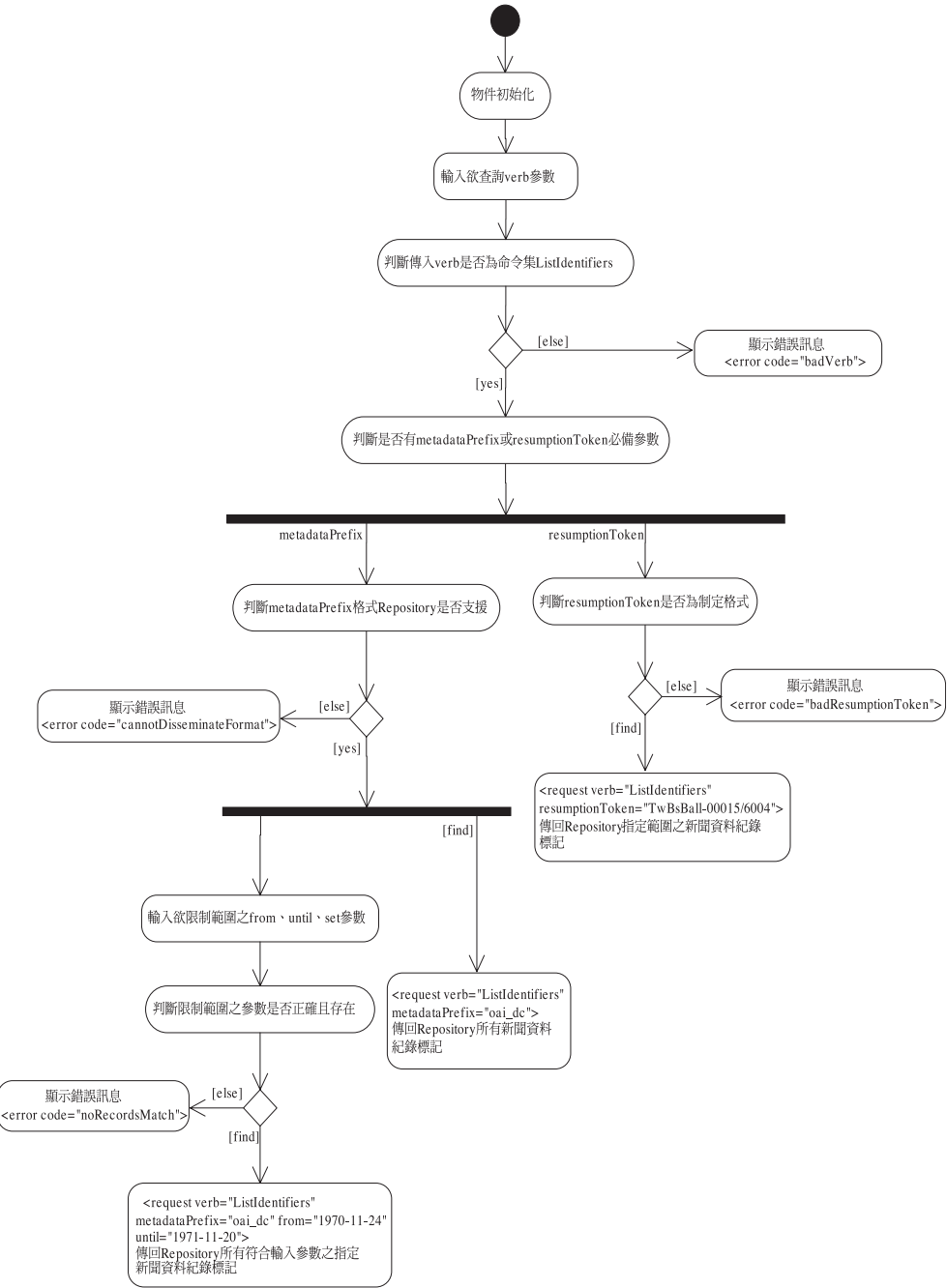
圖7 ListIdentifiers活動圖
