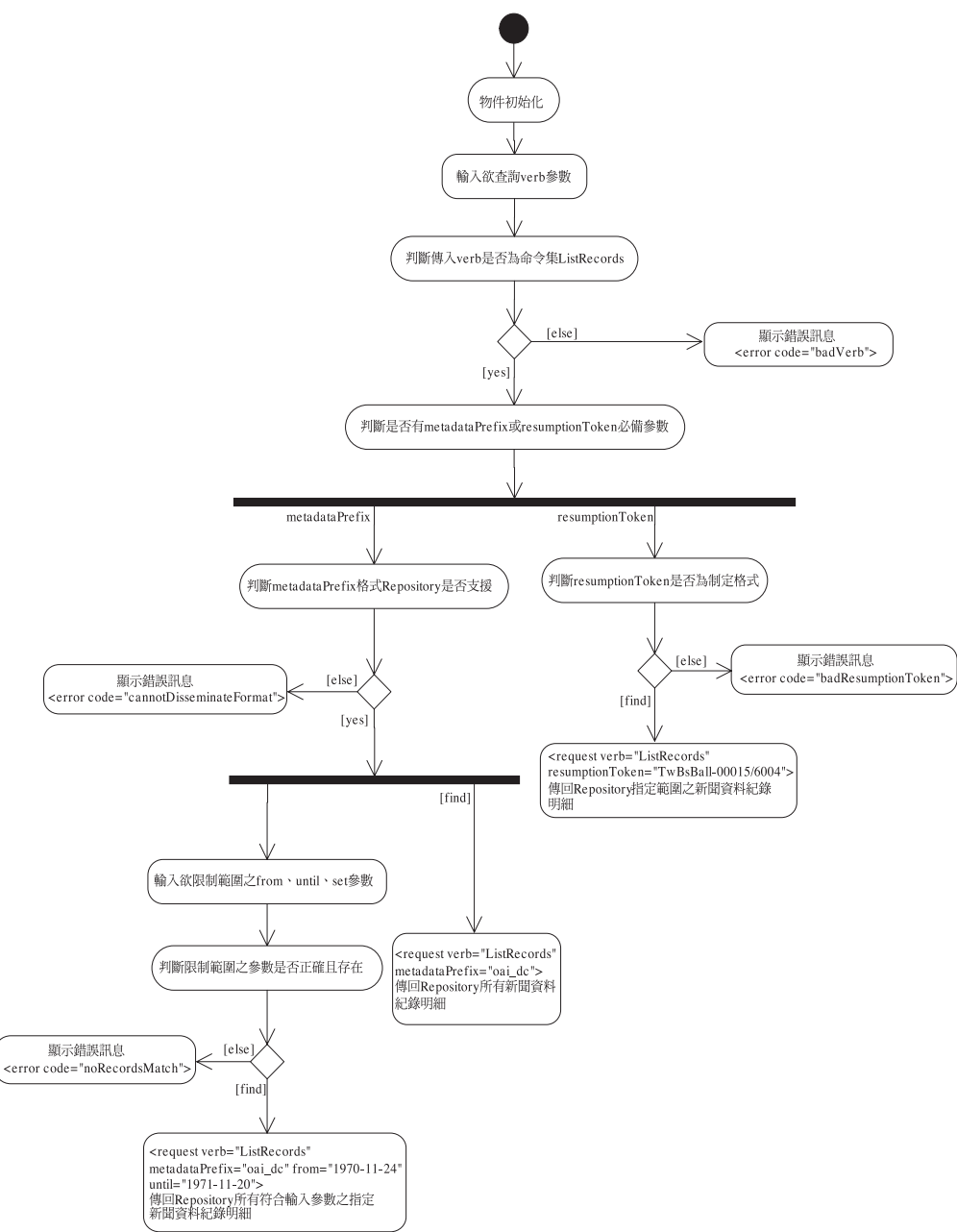
圖8 ListRecords活動圖
