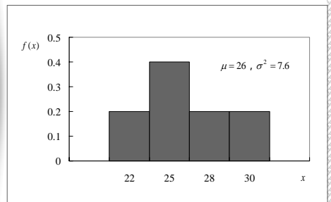
圖9.8 展示小姐月薪的母體機率分配
