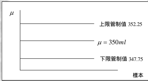
圖9.16 品質管制圖
