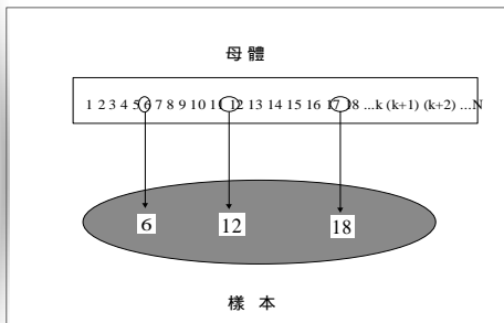
圖9.20 系統抽樣法
