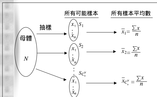
圖9.9 樣本平均數的抽樣分配
