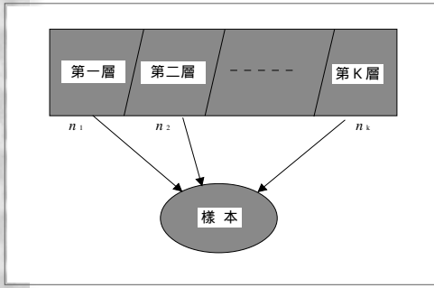
圖9.18 分層抽樣方法 - 比例抽樣
