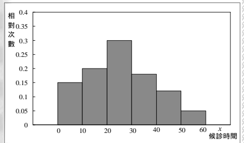
圖9.1 等待看牙時間(母體)
