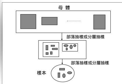
圖9.22 分段抽樣法
