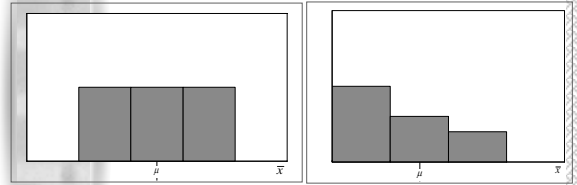
圖9.20 中央極限定理 母體分配 母體分配
