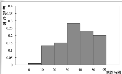
圖9.2 等待看牙時間(樣本1)
