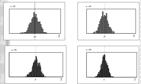
圖9.20 中央極限定理 (續)
