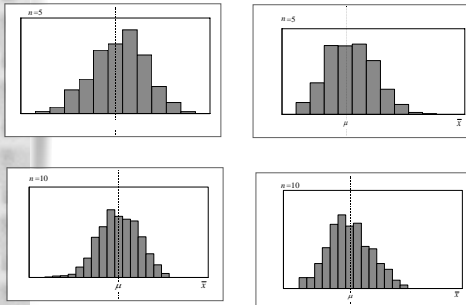
圖9.20 中央極限定理 (續)
