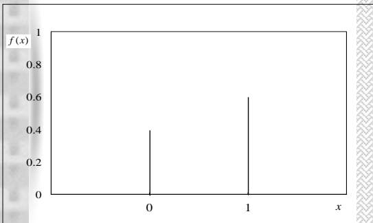
圖9.17 點二項分配
