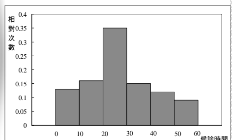
圖9.3 等待看牙時間(樣本2)
