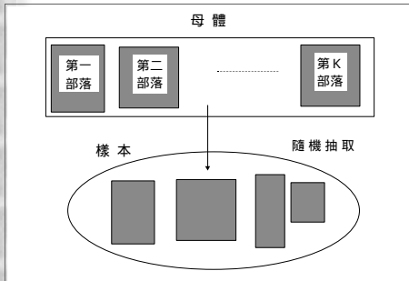
圖9.19 部落抽樣法
