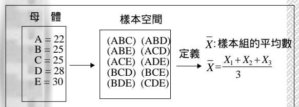
圖9.10 展示接待小姐月薪的抽樣
