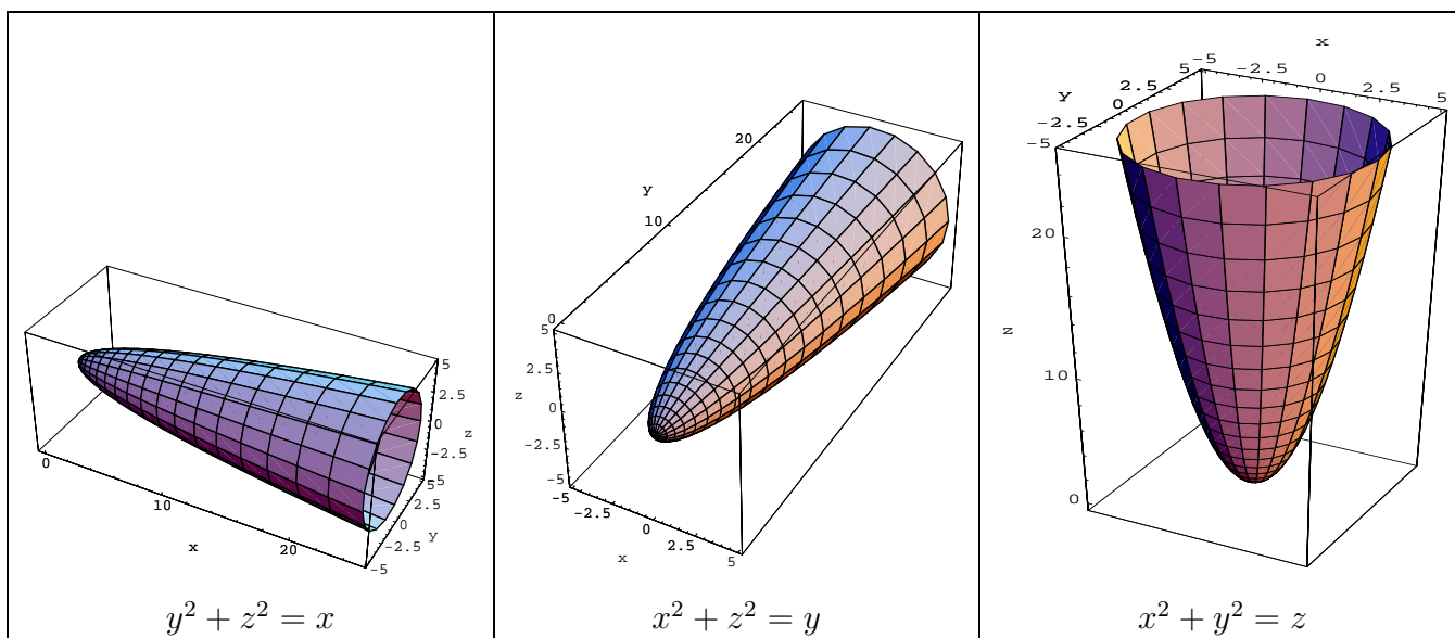
Paraboloids 拋物面
