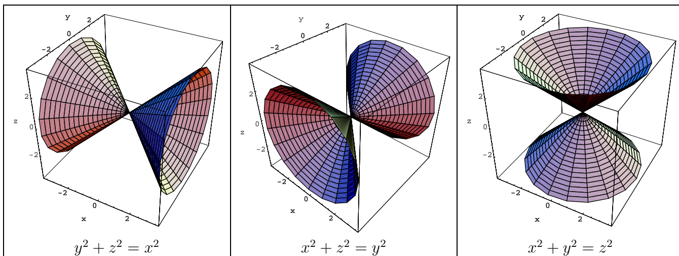
Cones 錐面
