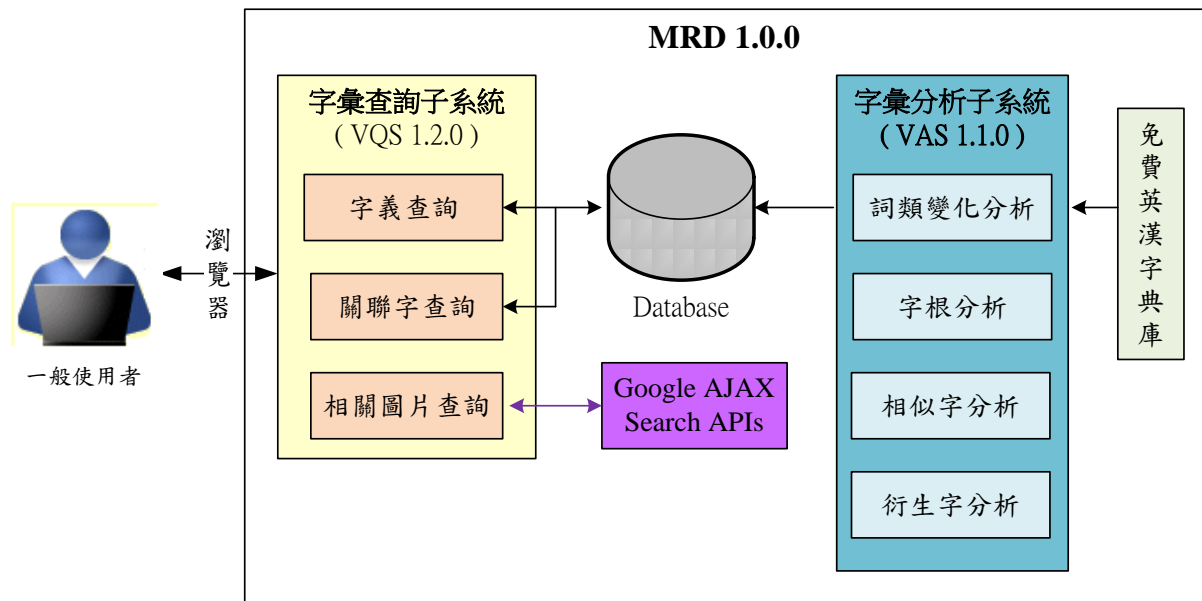
Figure 1. Mr. Root 線上英漢字典 2.0 系統架構圖
